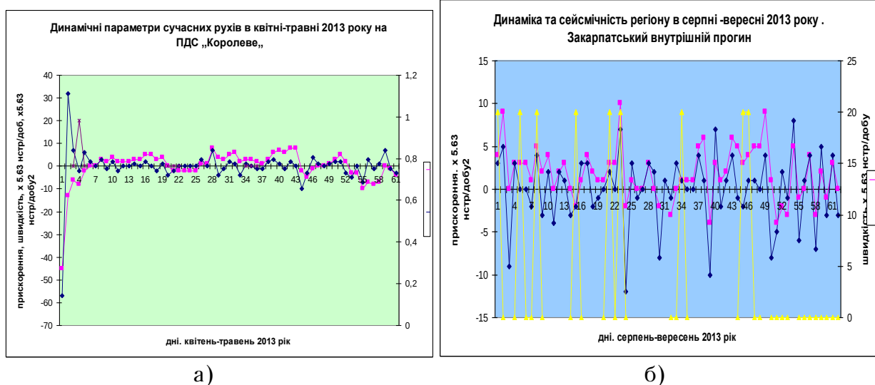
Рис.2. а) Динамічні параметри сучасних рухів земної кори на ПДС „Королеве,, за квітень-травень 2013 року та місцева сейсмічність; б) Динаміка та сейсмічність регіону в серпні-вересні 2013 року в Закарпатському внутрішньому прогині.
