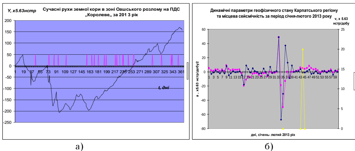
Рис. 1. а) Сучасні рухи земної кори на ПДС „Королеве„ за 2013 рік. Червоні вертикальні лінії вказують час реєстрації місцевих землетрусів; б) Динамічні параметри геофізичного стану Карпатського регіону та місцева сейсмічність за період січня-лютого 2013 року.
