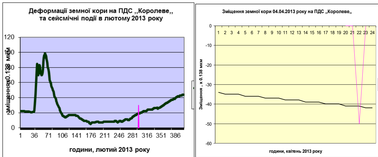
Рис.3. а) Коливання земної кори на ПДС „Королеве,, в лютому 2013 року та місцевий землетрус (13.02.2013 року); б) Зміщення земної кори на ПДС „Королеве,, в 04.04.2013 року, та час реєстрації місцевого землетрусу в Хустському районі.
