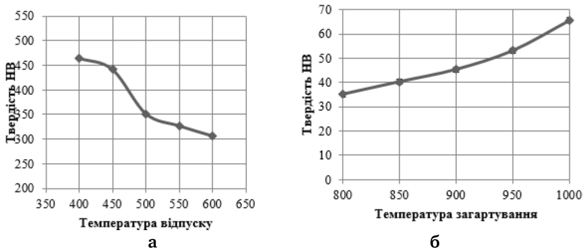
Рис. 1. Графік зміни твердості зразків залежно від температури відпуску та загартування а – кільце з чавуну ВЧ-50, б – масловідбивач зі сталі 40X
