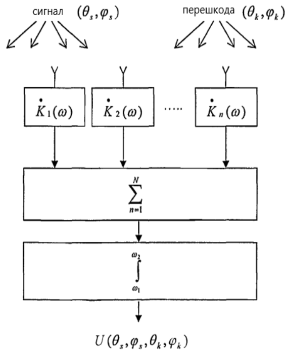
Рисунок 1 – Функціональна схема просторово-частотної обробки ШП сигналу
